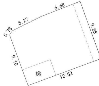
三幢三层平面图
