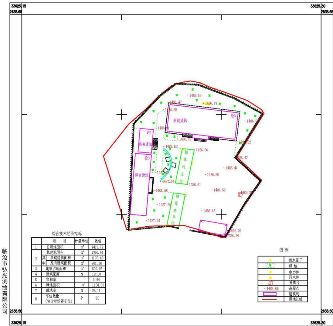
临沧市公安局临翔分局马台毒品检查站建设项目规划竣工验收平面图
