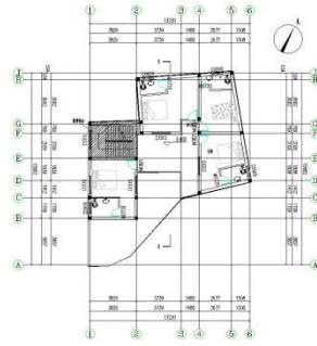
图四：四层平面图 1:101
