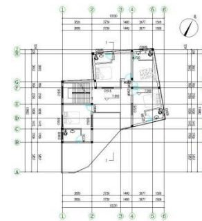
图七：七层平面图 1:101
