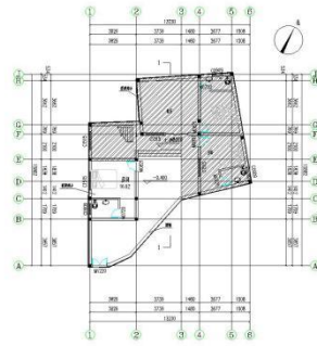
图一：一层平面图 1:101
