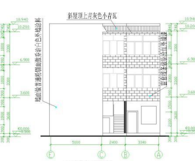
左侧立面图 1:100
