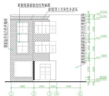
正立面图 1:100
