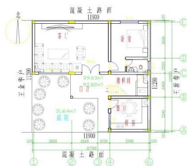
一层平面图 1:100
