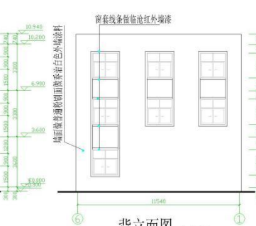
背立面图 1:100
