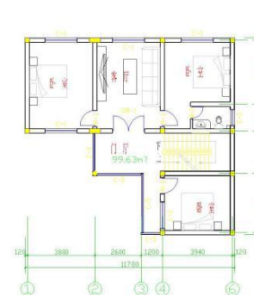
二层平面图 1:100
