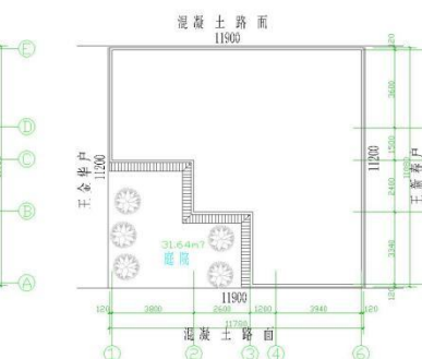
屋顶平面图 1:100
