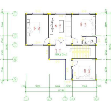
三层平面图 1:100
