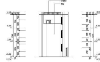
⑤—⑥轴立面图 1:100
