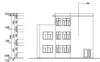
①—②轴立面图 1:100
