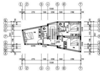
二层平面图 1:100 本层建筑面积70.03m 2
