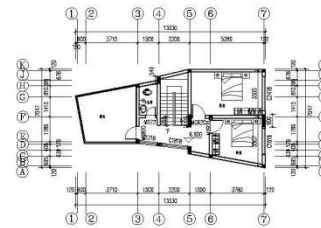
三层平面图 1:100 本层建筑面积54.55m 2
