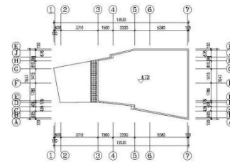
屋顶平面图 1:100
