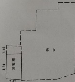
屋顶层平面图
