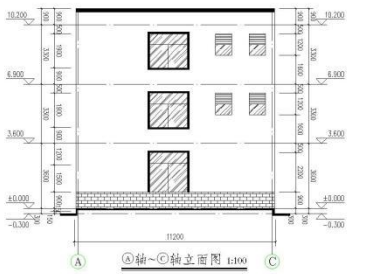
A-A轴~A-A轴立面图 1:100
