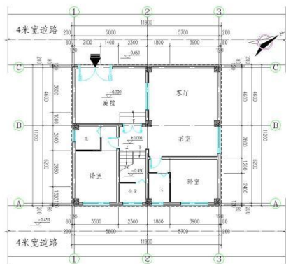
总平面布置图 1:400
