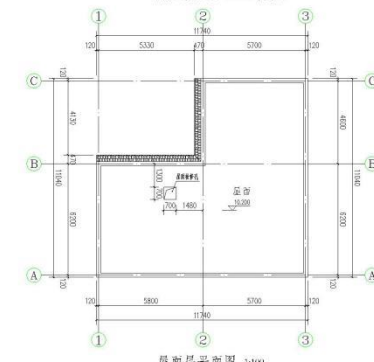
屋面平面图 1:100
