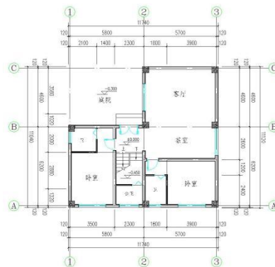
三层平面图 1:100
