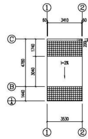
屋面层平面图 1:200
