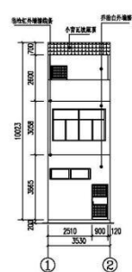
1~2立面图 1:200
