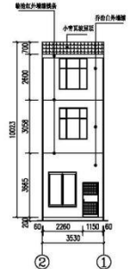
2~1立面图 1:200
