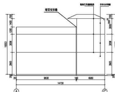
A~C立面图 1:200
