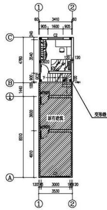
二层平面图 1:200
