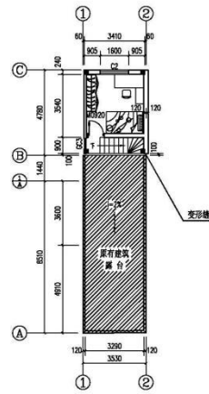
三层平面图 1:200
