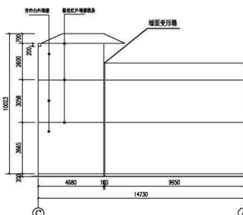
0~A立面图 1:200
