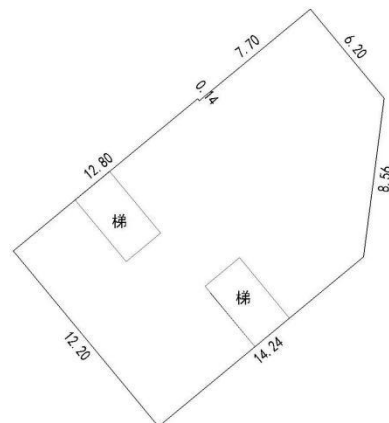
一幢四层平面图
