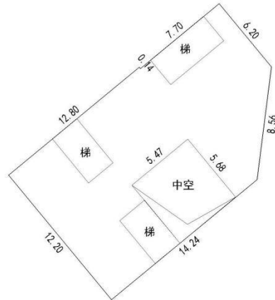
一幢三层平面图
