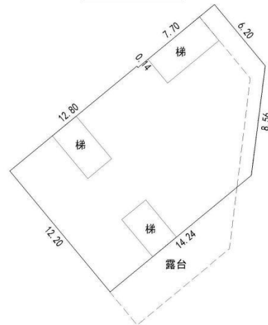
一幢二层平面图
