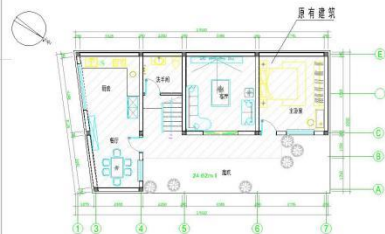
原建一层平面图 1:100
