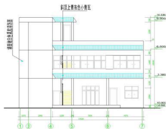
正立面图 1:100
