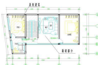
二层平面图 1:100
