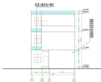
右侧立面图 1:100
