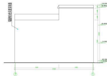
背立面图 1:100
