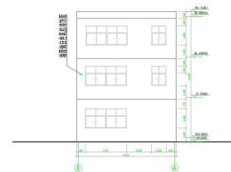
左侧立面图 1:100
