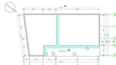
屋顶平面图 1:100
