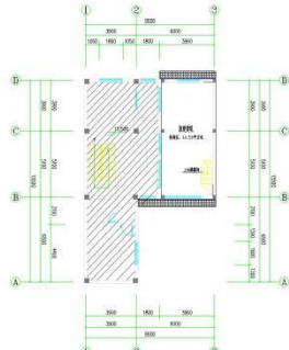
四层平面图 1:100 本层建筑面积: 85.57平方米 卫生间地坪标高: 34.500 卫生间地坪标高: 10.450
