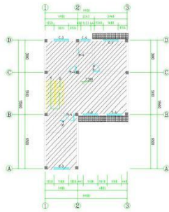
三层平面图 1:100 本层建筑面积: 122.16平方米 卫生间地坪标高: 7.150
