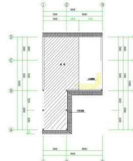
五层平面图 1:100
