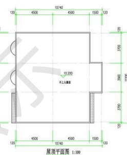
屋顶平面图 1:100
