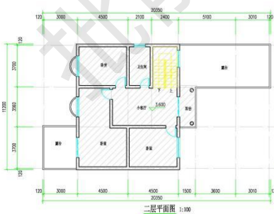
二层平面图 1:100 本层建筑基底为108.84平方米 其中：住宅部分
