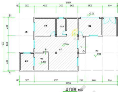
一层平面图 1:100 本层建筑基底为133.12平方米 其中：裙房部分
