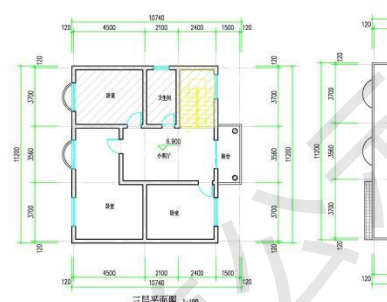
三层平面图 1:100 本层建筑基底为108.84平方米 其中：住宅部分为43.53平方米 其中：内庭部分为65.31平方米 其中：原有建筑
