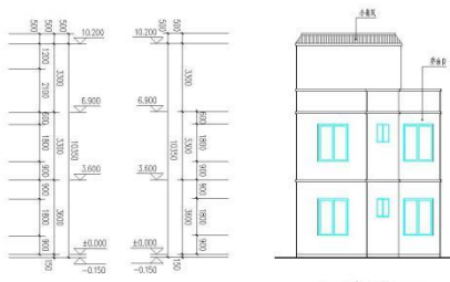
①-②轴立面图 1:100
