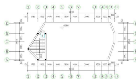
三层平面 1:100 本层建筑面积: 12.75m 2
