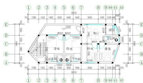
二层平面 1:100 本层建筑面积: 93.34m 2
