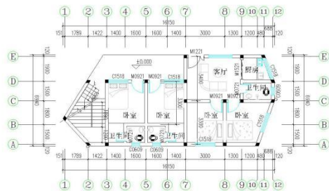
一层平面 1:100 本层建筑面积: 93.34m 2 总建筑面积: 199.43m 2
