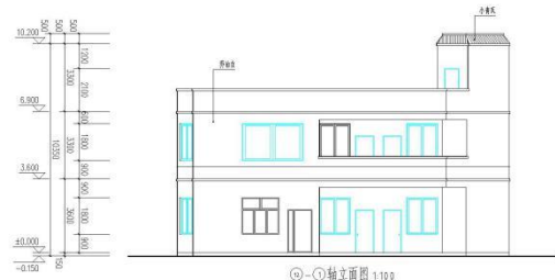
③-④轴立面图 1:100
