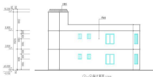
①-④轴立面图 1:100
