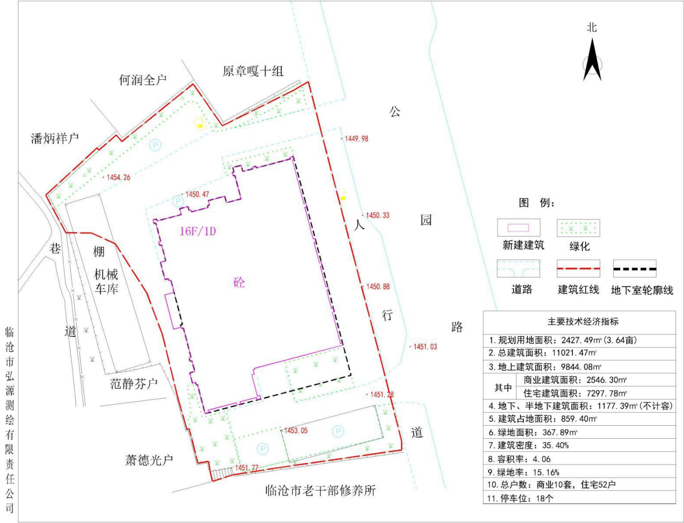
都市明珠商住小区建设项目规划竣工实测平面图
