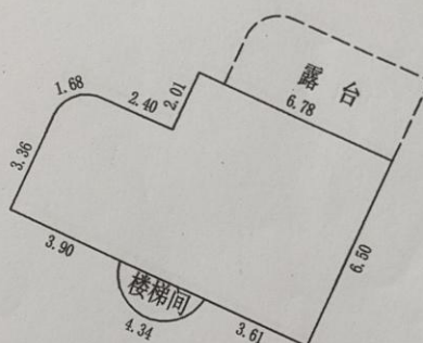
一幢二层平面图
