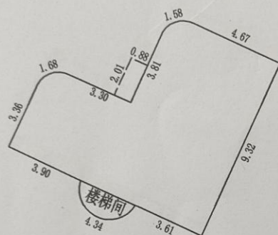
一幢一层平面图
