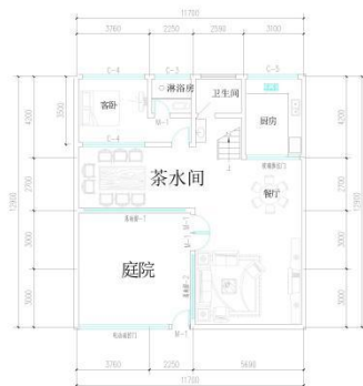
一层平面图
