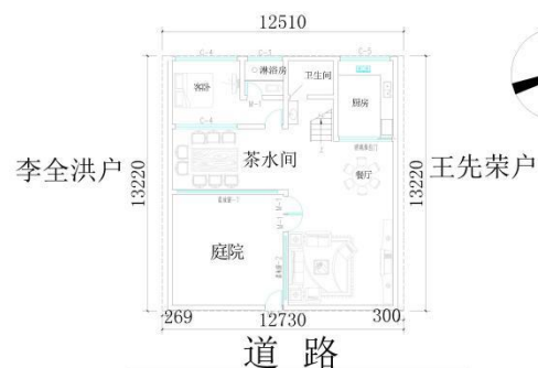
一层平面图
