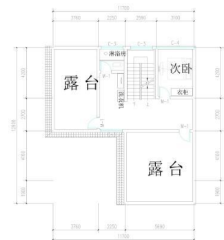
三层平面图
