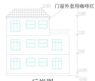
后视图
