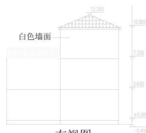
右视图
