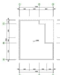
一层平面图 (1:100)
