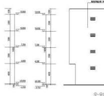
⑤-⑥立面图 (1:100)
