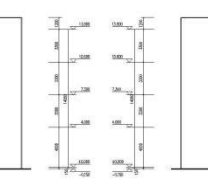
⑦-⑧立面图 (1:100)
