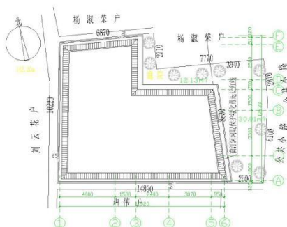
屋顶平面图 1:100
