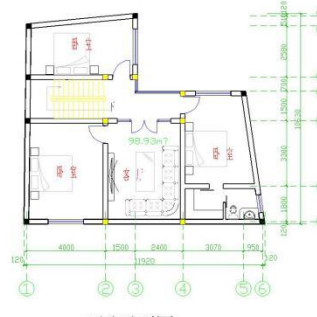
三层平面图 1:100
