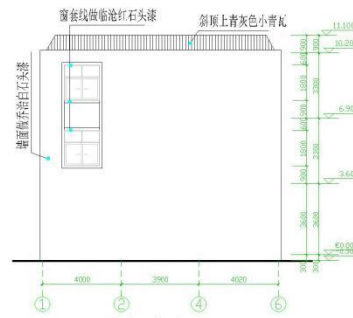
背立面图 1:100
