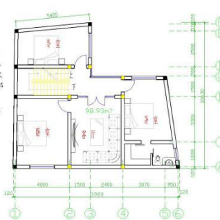
二层平面图 1:100
