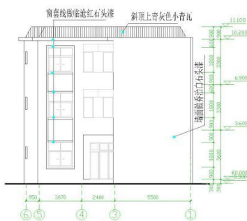
正立面图 1:100
