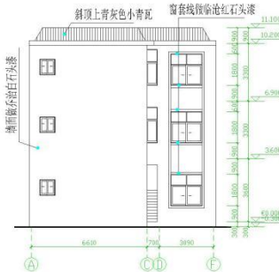
右侧立面图 1:100
