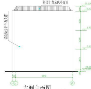
左侧立面图 1:100
