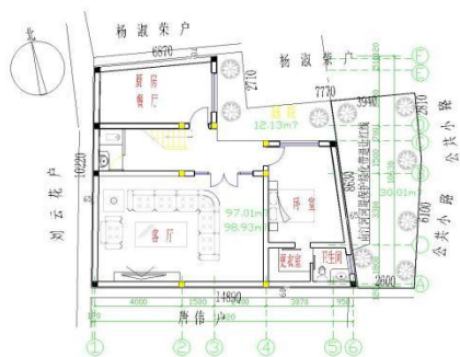
一层平面图 1:100
