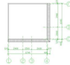
屋顶平面图 1:100
