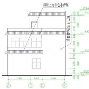
右侧立面图 1:100
