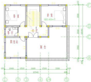
二层平面图 1:100
