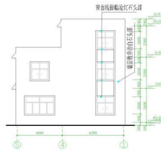
背立面图 1:100
