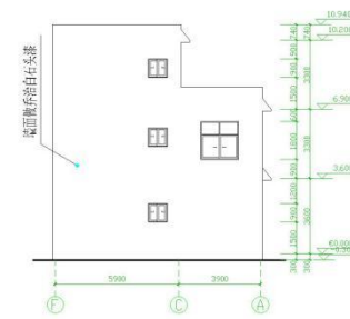
左侧立面图 1:100
