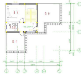
三层平面图 1:100
