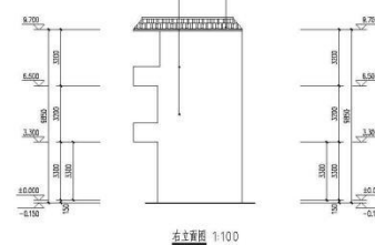
右后立面图 1:100
