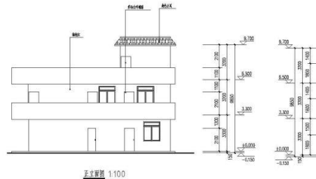
正面立面图 1:100
