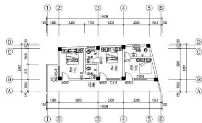
二层平面图 1:100 二层建筑面积: 67.82平方米
