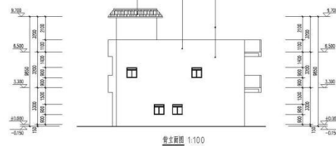
背面立面图 1:100
