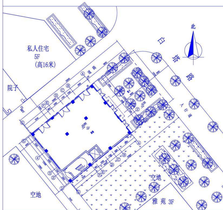
总平面图
