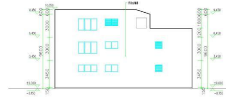
东立面图 1:100
