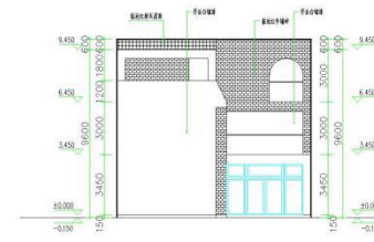
左立面图 1:100
