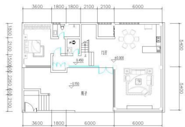
一层平面图 1:100
