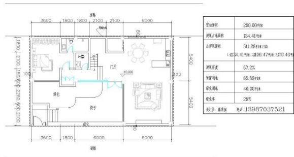
总平面图 1:100
