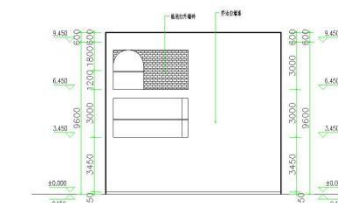
右立面图 1:100
