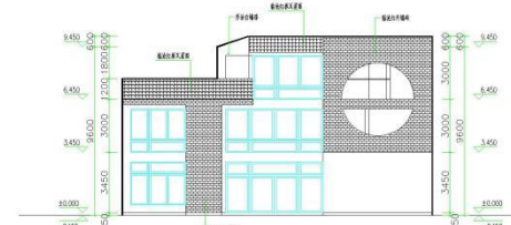
左立面图 1:100
