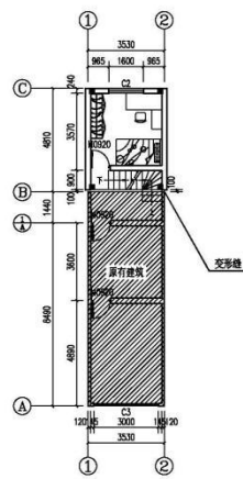
二层平面图 1:200
