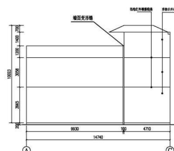
①~③立面图 1:200
