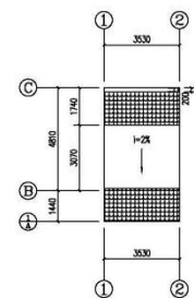
屋面层平面图 1:200
