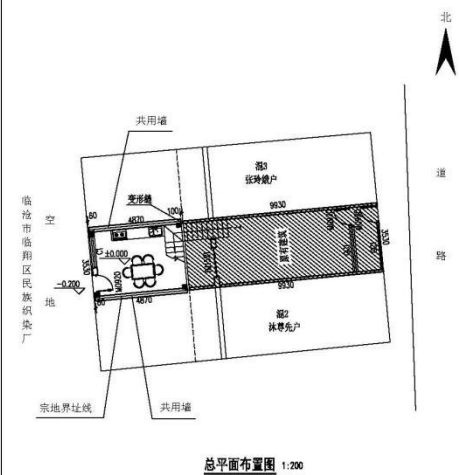
总平面布置图 1:200
