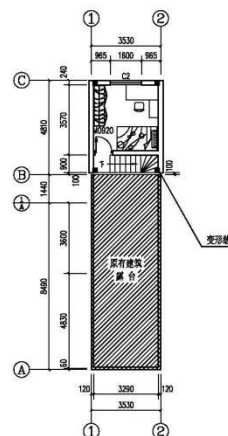
三层平面图 1:200
