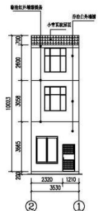
②~①立面图 1:200
