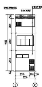
①~②立面图 1:200
