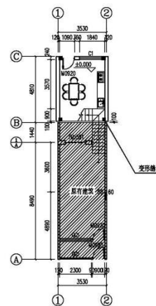
一层平面图 1:200
