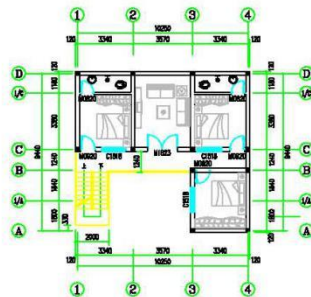
二层平面图 1:250
