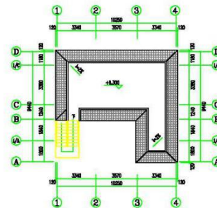
屋面平面图 1:250
