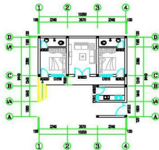
一层平面图 1:250
