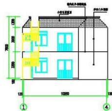
①~④立面图 1:250
