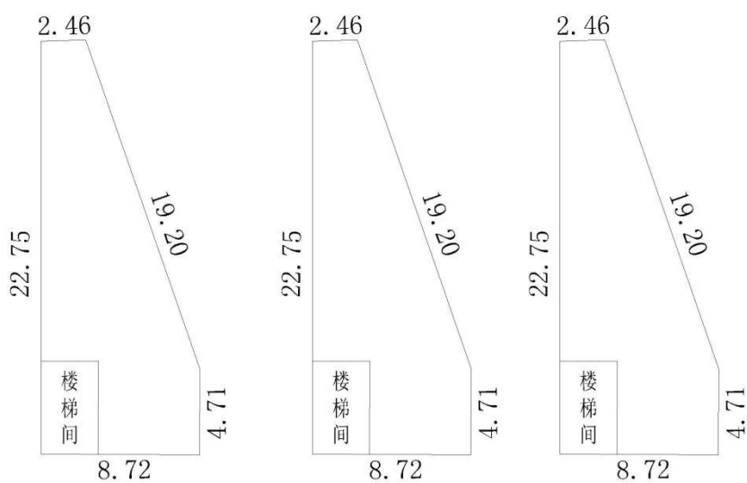
1幢一层平面图
