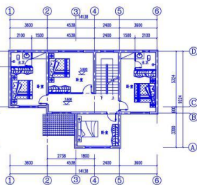
二层平面图 1:100
