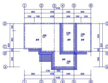
屋顶平面图 1:100
