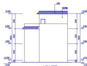
右侧立面图 1:100
