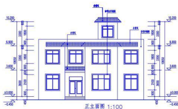
正立面图 1:100
