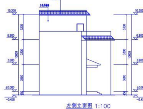
左侧立面图 1:100
