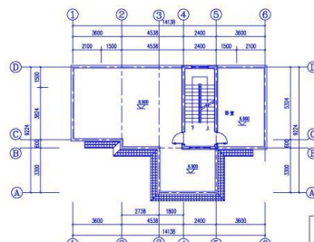
三层平面图 1:100
