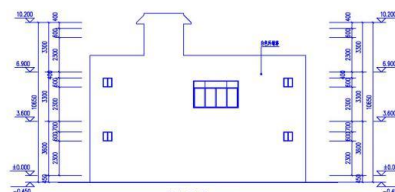
背立面图 1:100
