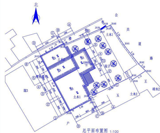
总平面布置图 1:100
