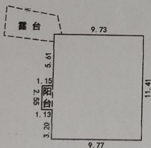
三层平面图
