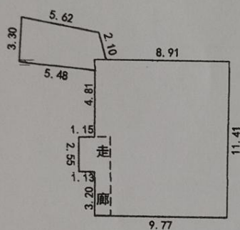
一层平面图
