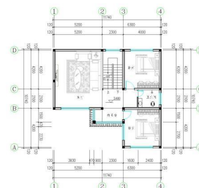
八层平面图 1:100
