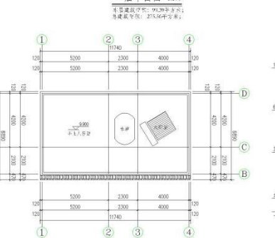
五层平面图 1:100
