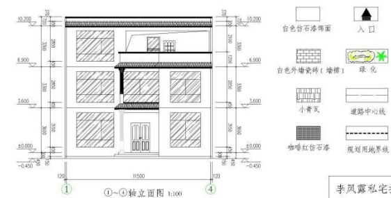
①~①轴立面图 1:100
