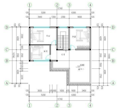
一层平面图 1:100
