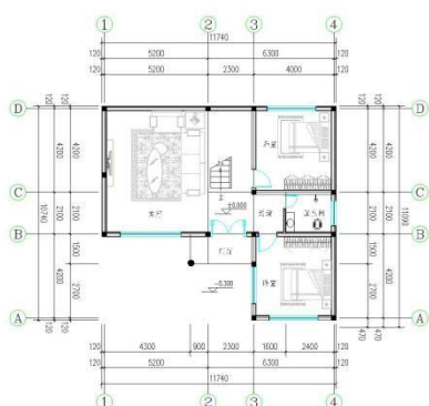
四层平面图 1:100
