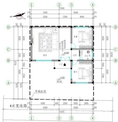
总平面布置图 1:100
